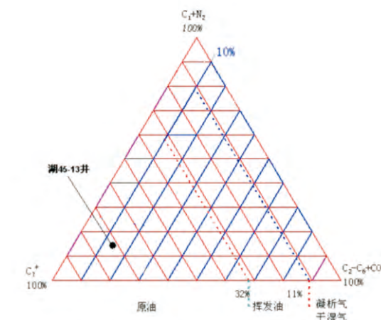
图2 油气藏流体类型三角相图
